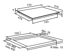
Tezgah üstü montaj ölçüsü
