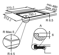
Tezgaha sıfır montaj ölçüsü
