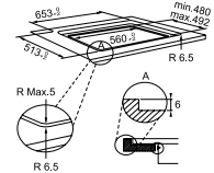
Tezgaha sıfır montaj ölçüsü
