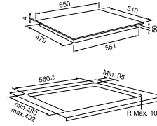
Tezgah üstü montaj ölçüsü
