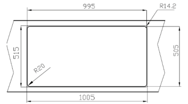
Tezgaha sıfır montaj ölçüsü
